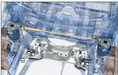
パフォーマンスダンパー®(フロント)
