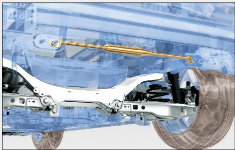
パフォーマンスダンパー®(リヤ)
