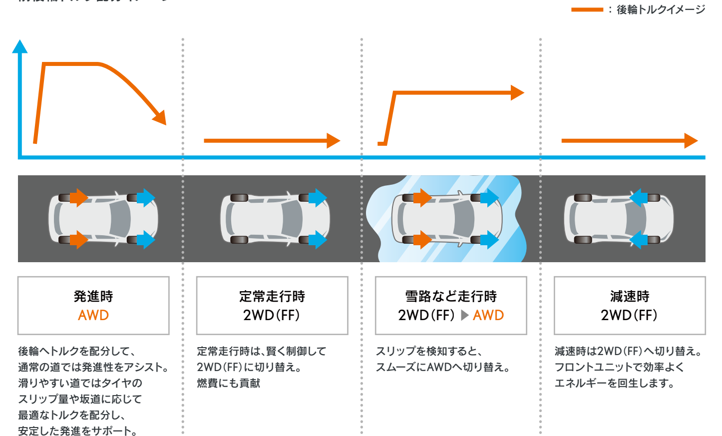
前後輪トルク配分イメージ
