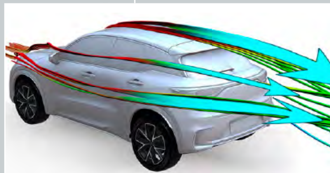
①ルーフ形状・門型スポイラー・リヤコンビネーションランプにより車両後方への流れを適正化しCd値低減・優れた直進安定性を実現
