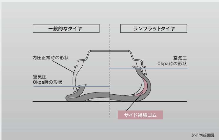
タイヤ断面図
