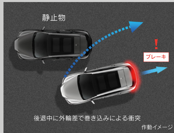
パーキングサポートブレーキ(周囲静止物) [PKSB]
